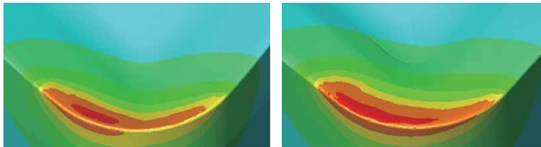
SQ Chipbreaker
